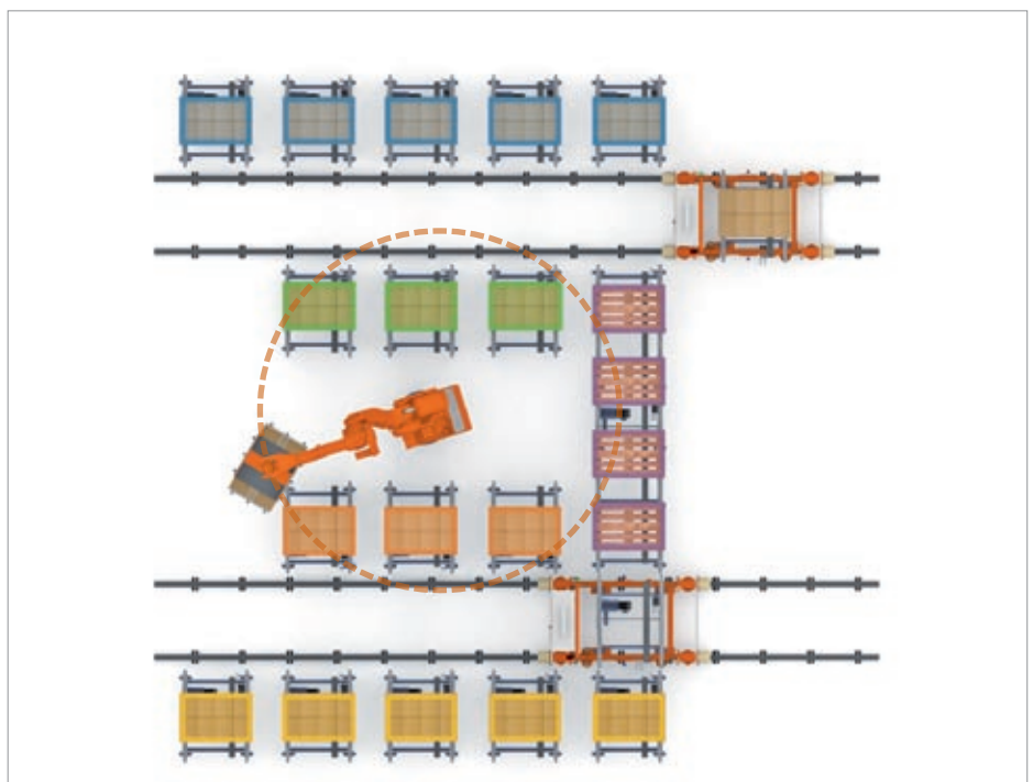
Schéma de fonctionnement du système de picking automatique par robot dépalettiseur.
